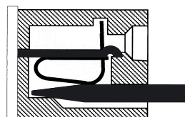
Fig. 3 Sezione A-A in fig. 2
